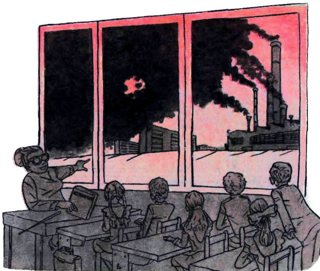
— А вот как примерно, дети, выглядит солнечное затмение. Рисунок В. ТИЛЬМАНА.
